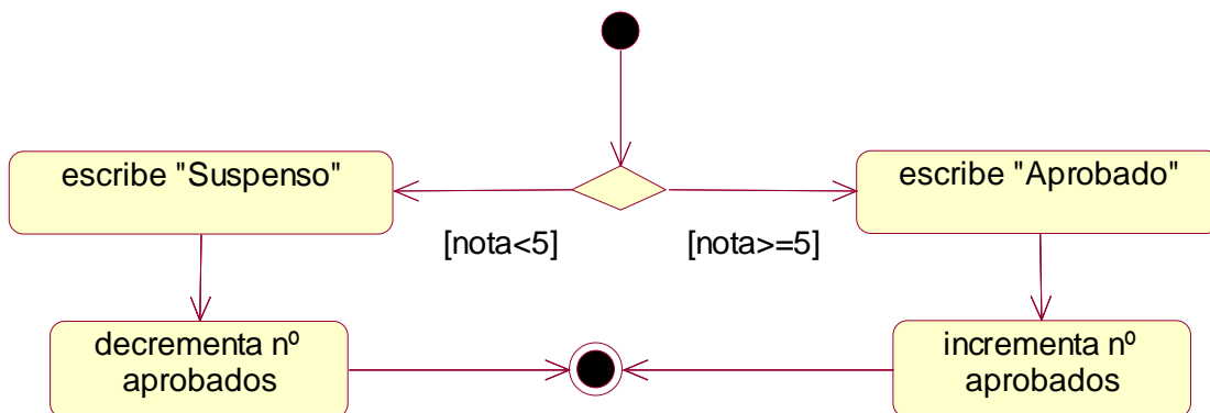
Ilustración 3-2, Diagrama de actividad de una instrucción if doble
